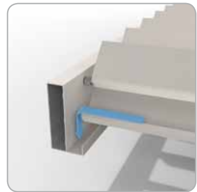
Abflussrinne
